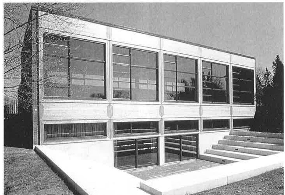
Renovierte Südwestfassade
