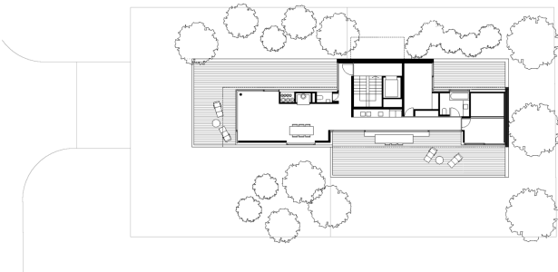
Dachgeschoss
