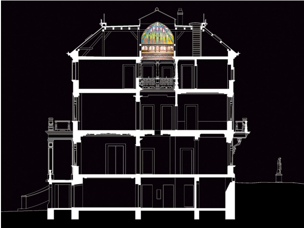
Villa Querschnitt
