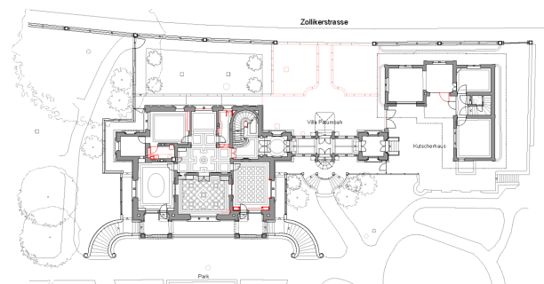
Erdgeschoss
