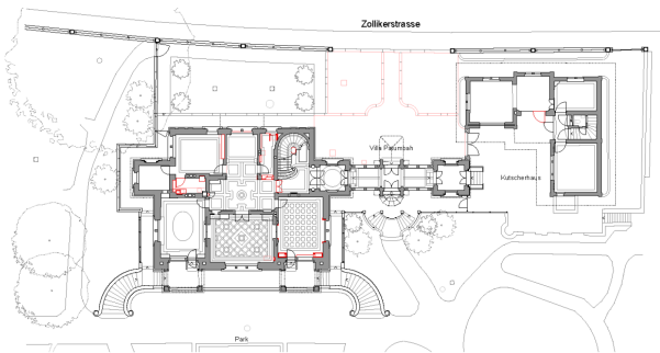
Erdgeschoss
