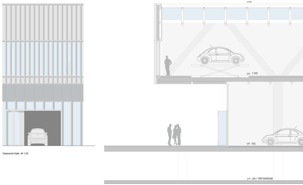
Teilansicht und -Schnitt Halle
