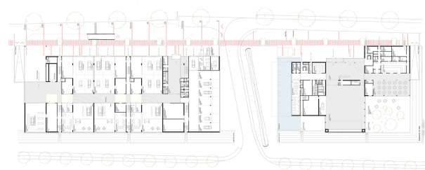
Erdgeschoss
