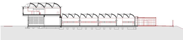
Längsschnitt
