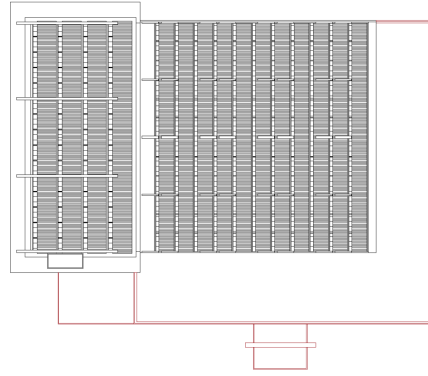
Dachaufsicht
