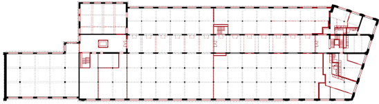
1. Obergeschoss
