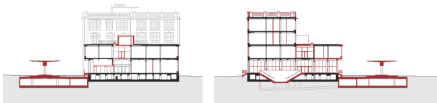
Querschnitte
