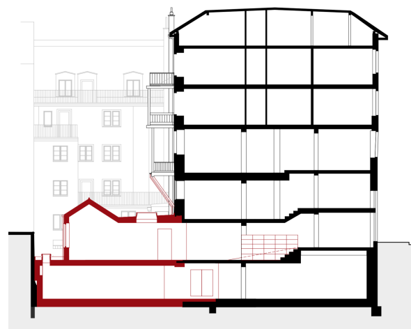
Längsschnitt
