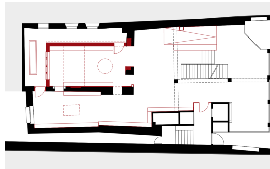
Erdgeschoss
