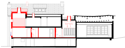
Längsschnitt
