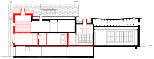
Längsschnitt
