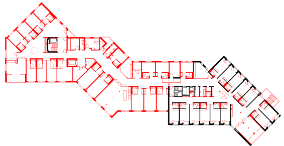
3. Obergeschoss
