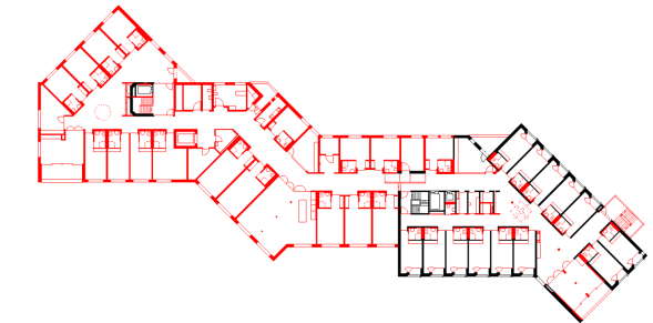
3. Obergeschoss
