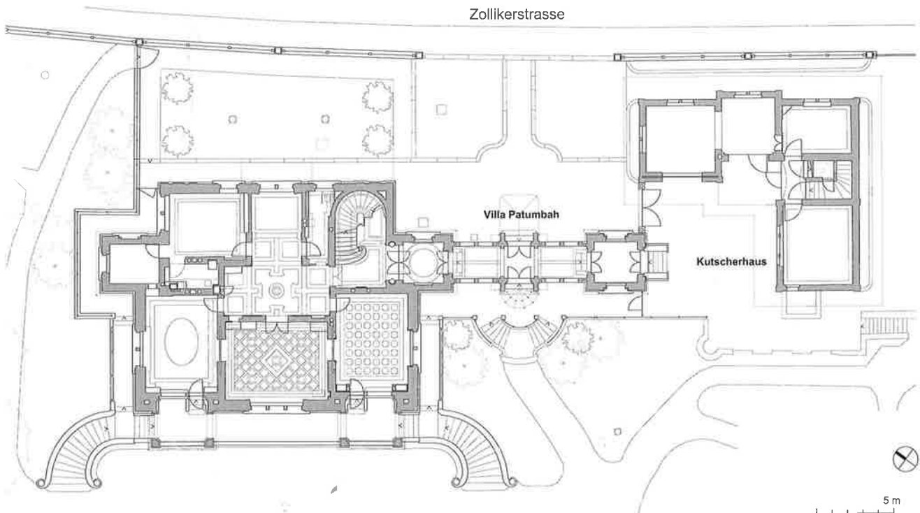
Erdgeschoss Rez-de-chaussée
