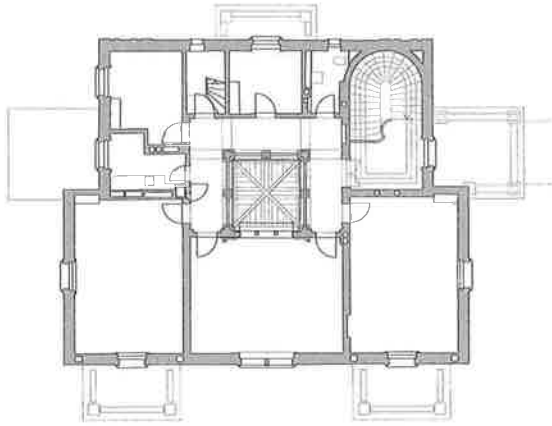
2. Obergeschoss 2 e étage
